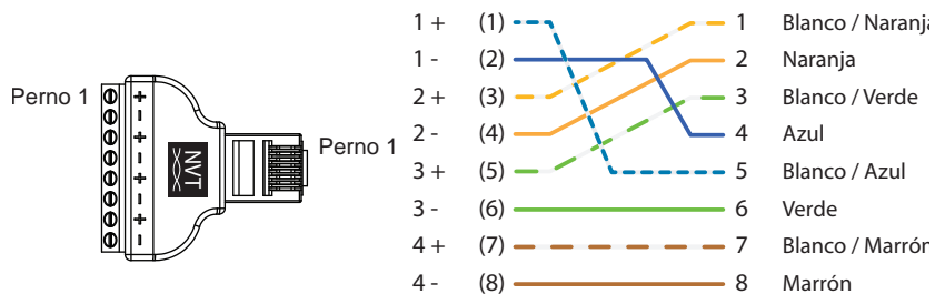
Tornillo del bloque de terminales canal pinout
